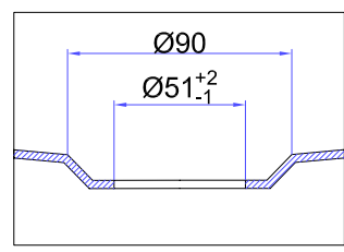
C-C
