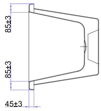
B-B
